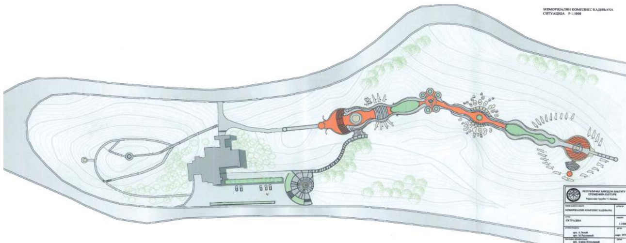
Меморијални комплекс Кадињача, ситуациони план
